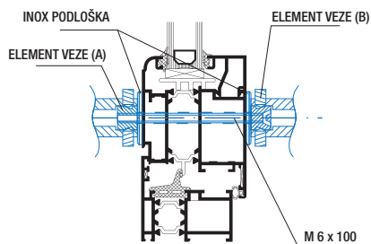
ravan prihvat
