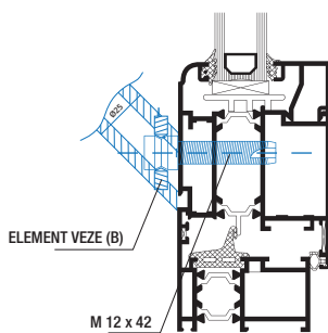
kosi prihvat
