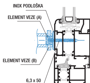
ravan prihvat
